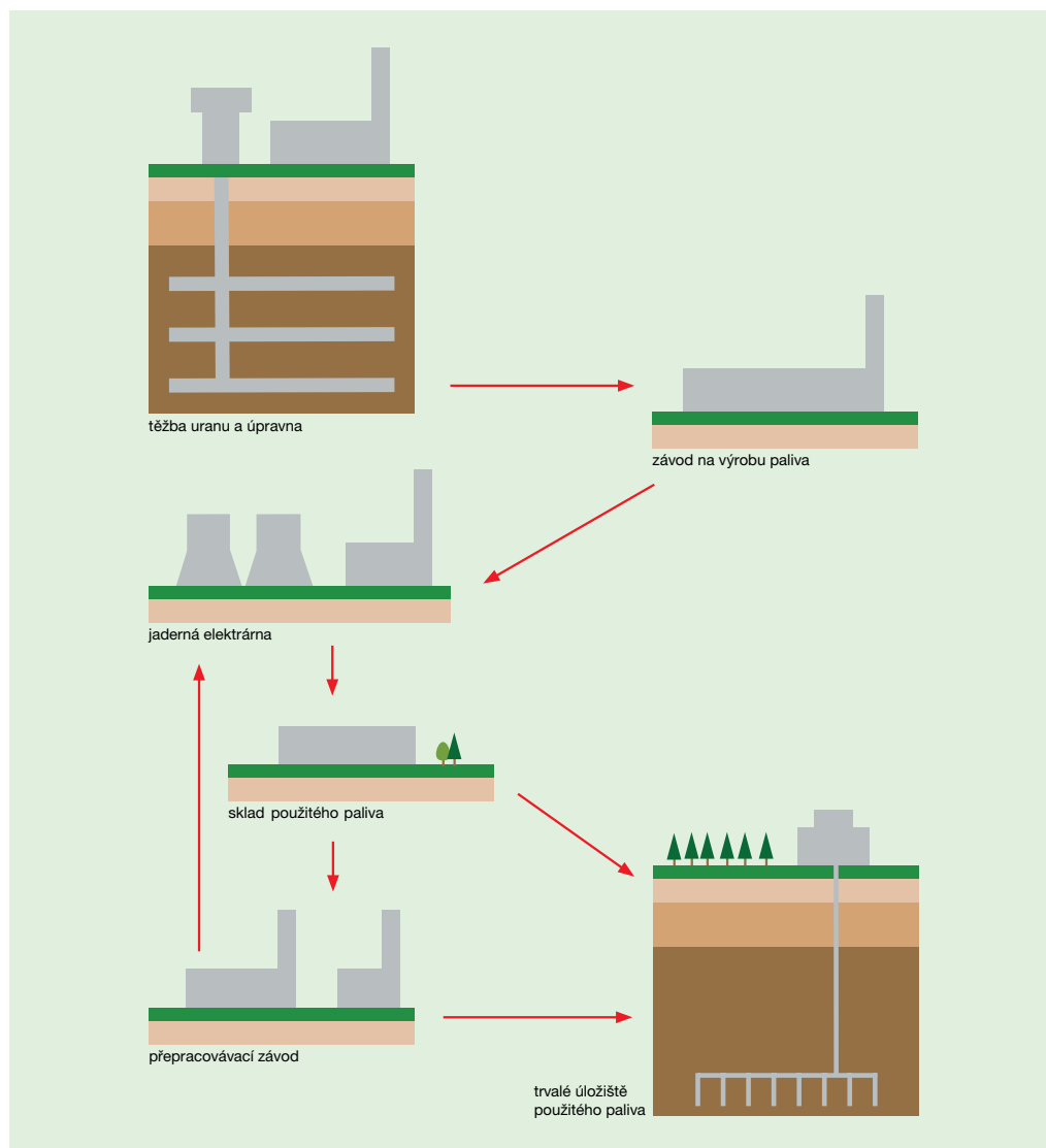
Schéma palivového cyklu jaderných elektráren. V České republice putuje použité palivo z elektrárny přímo do meziskladu.
